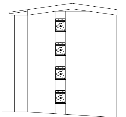
ZÁPADNÝ POHLAD
